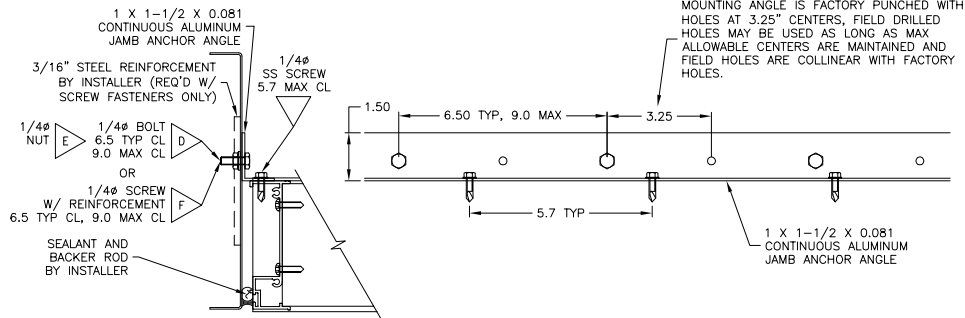
Ⓐ JAMB ANCHOR
