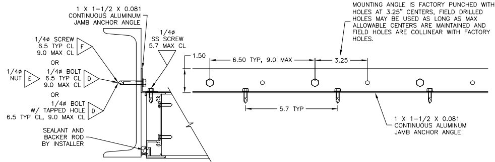
Ⓐ JAMB ANCHOR
